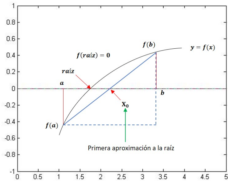
Figura 6: Establecimiento de la cuerda y obtención de la primera aproximación
