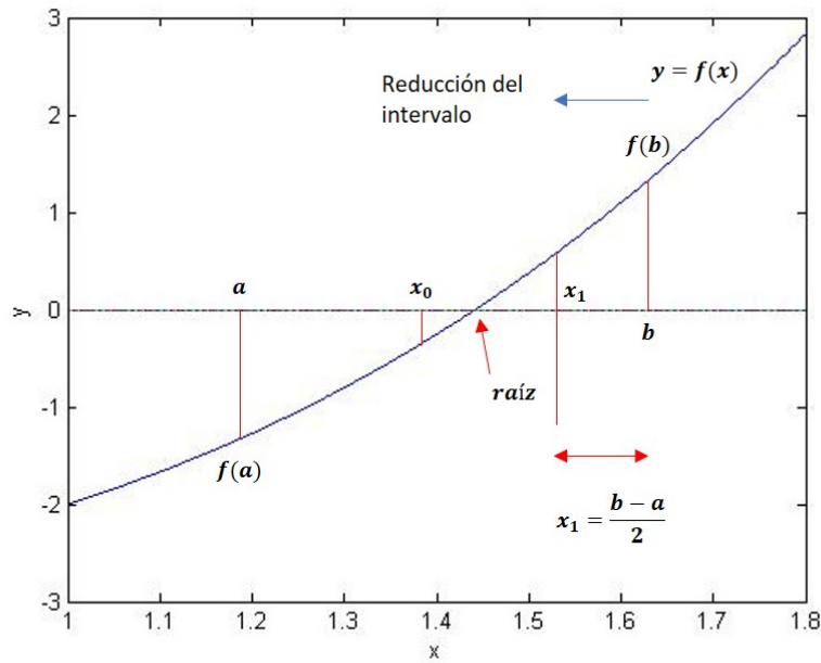
Figura 3: Intervalo reducido por la izquierda
