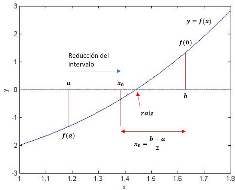
Figura 2: Intervalo reducido por la izquierda
