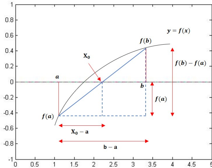
Figura 9: Triángulos semejantes a partir de la primera aproximación a la raíz
