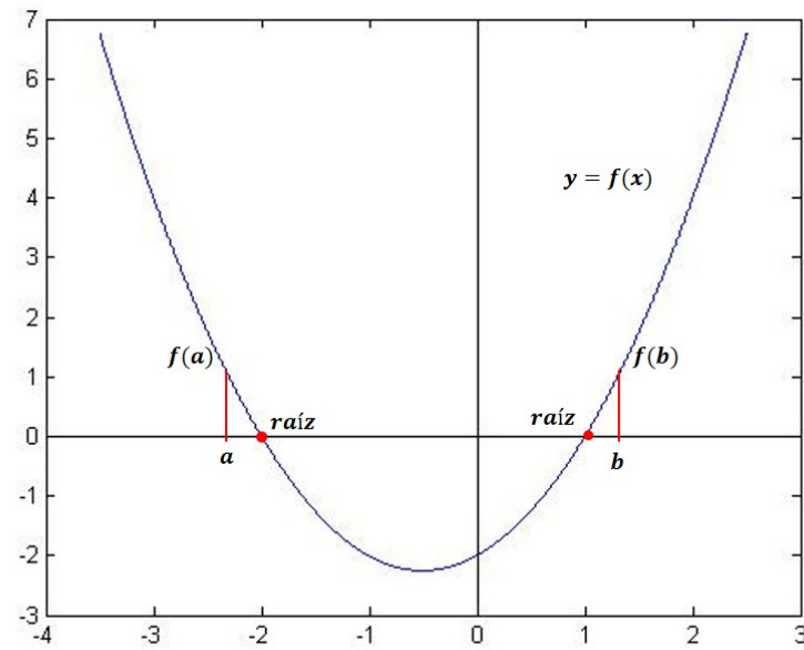
Figura 13: Raíces pares en la función
