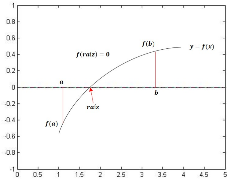
Figura 5: Intervalo [a, b] que atrapa una raíz
