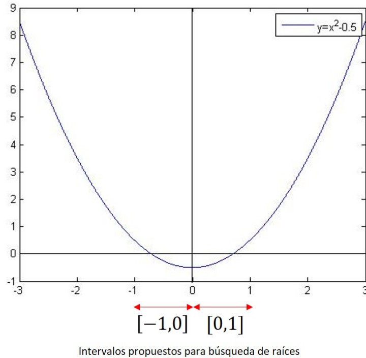
Figura 4: Intervalos iniciales de solución
