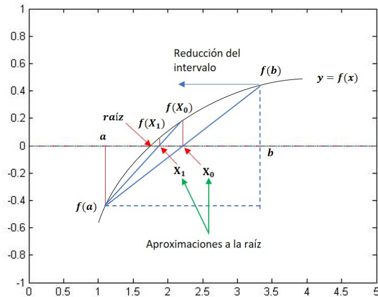
Figura 8: Obtención de las siguientes aproximaciones a la raíz
