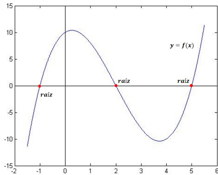
Figura 11: Total de raíces de la función
