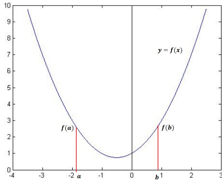
Figura 12: Función sin raíces reales
