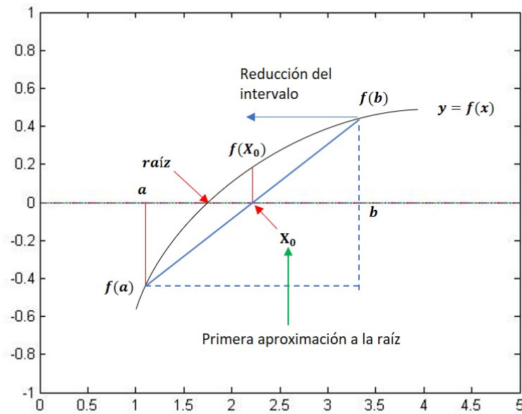
Figura 7: Reducción del intervalo que atrapa a la raíz
