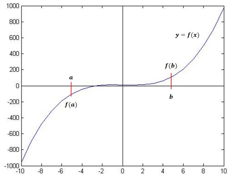
Figura 10: Intervalo que atrapa una raíz
