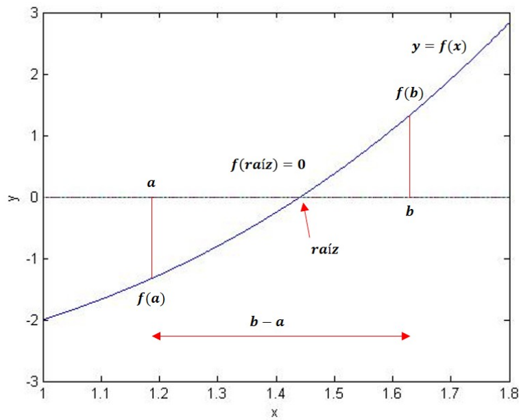
Figura 1: Intervalo [a, b] que atrapa una raíz
