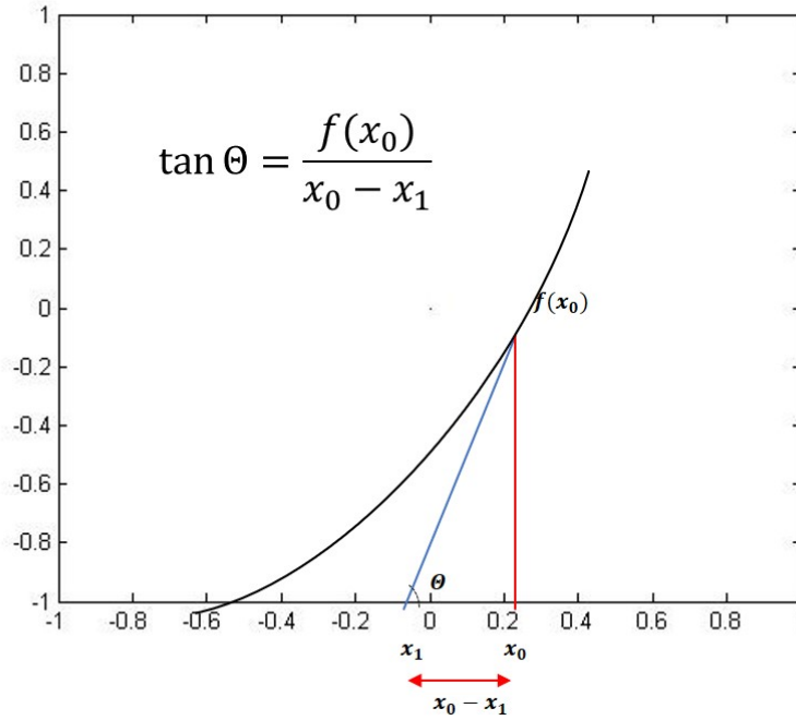
Figura 6: Obtención de la ecuación de recurrencia
