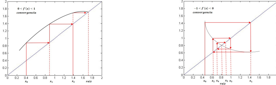
Figura 2: Casos de convergencia monotónica y oscilatoria
