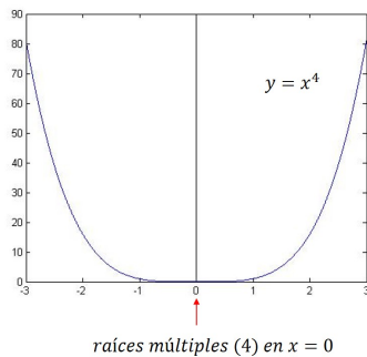
Figura 10: Cuatro raíces múltiples
