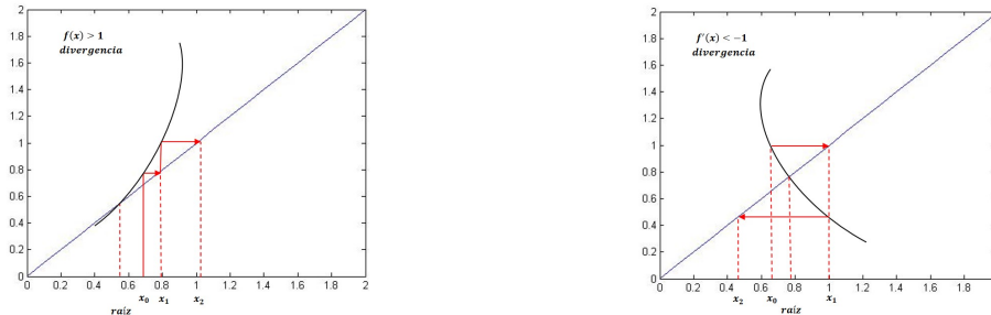
Figura 3: Casos de divergencia: monotónica y oscilatoria
