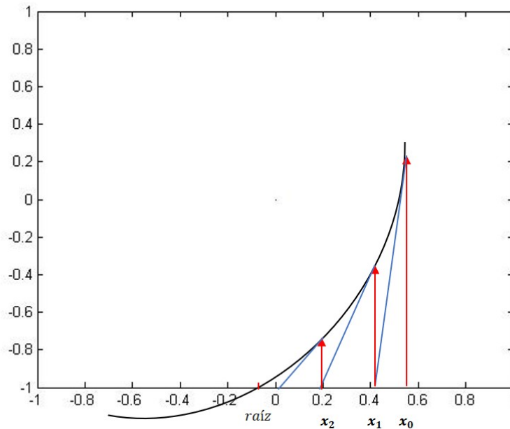
Figura 5: Interpretación geométrica del método Newton-Raphson
