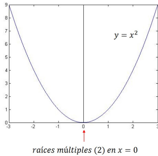
Figura 8: Dos raíces múltiples
