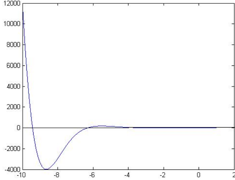
Figura 7: Ejemplo de aplicación
