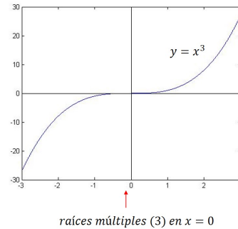
Figura 9: tres raíces múltiples
