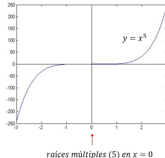
Figura 11: Cinco raíces múltiples
