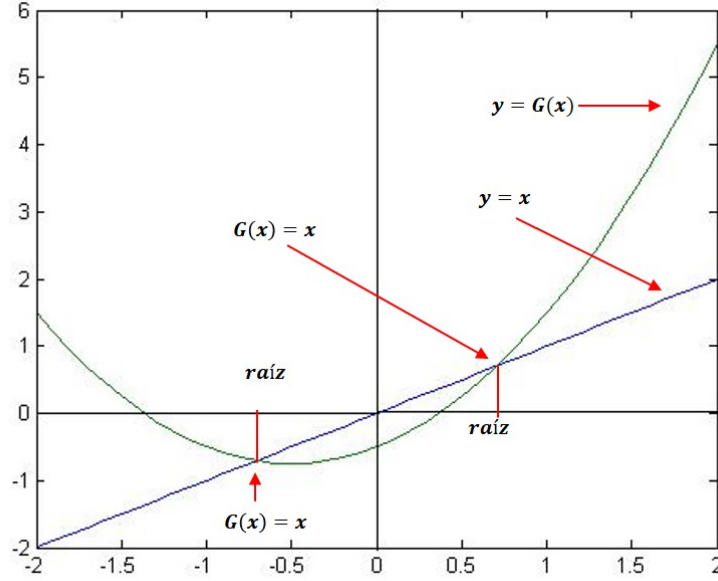
Figura 1: Interpretación geométrica del método de Aproximaciones sucesivas
